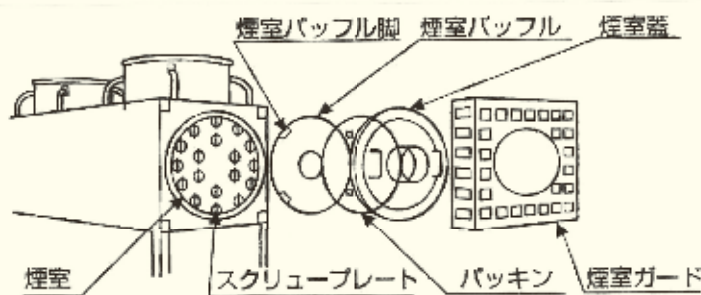
図2. 各部材名称（提供：ネポン(株)）
